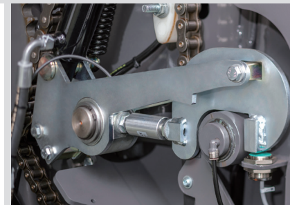
▲기계식 뒷문 잠금장치
