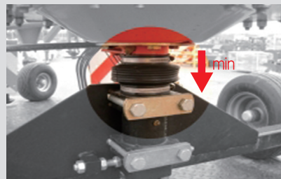
▲ 작업높이 조정
